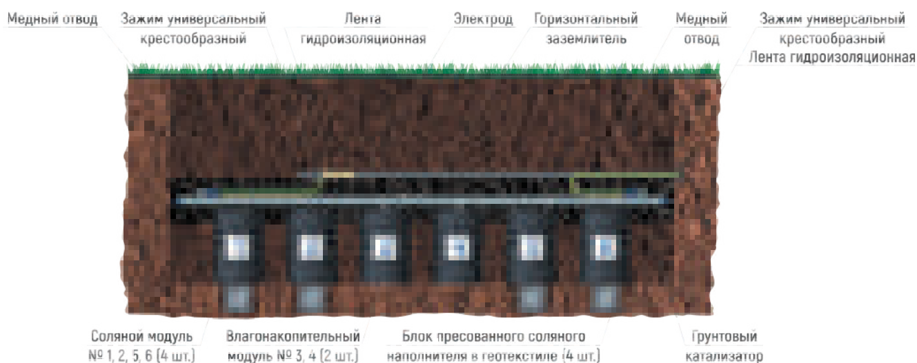
Рис. 7. Необслуживаемый активный соляной электрод «10 Ом»
